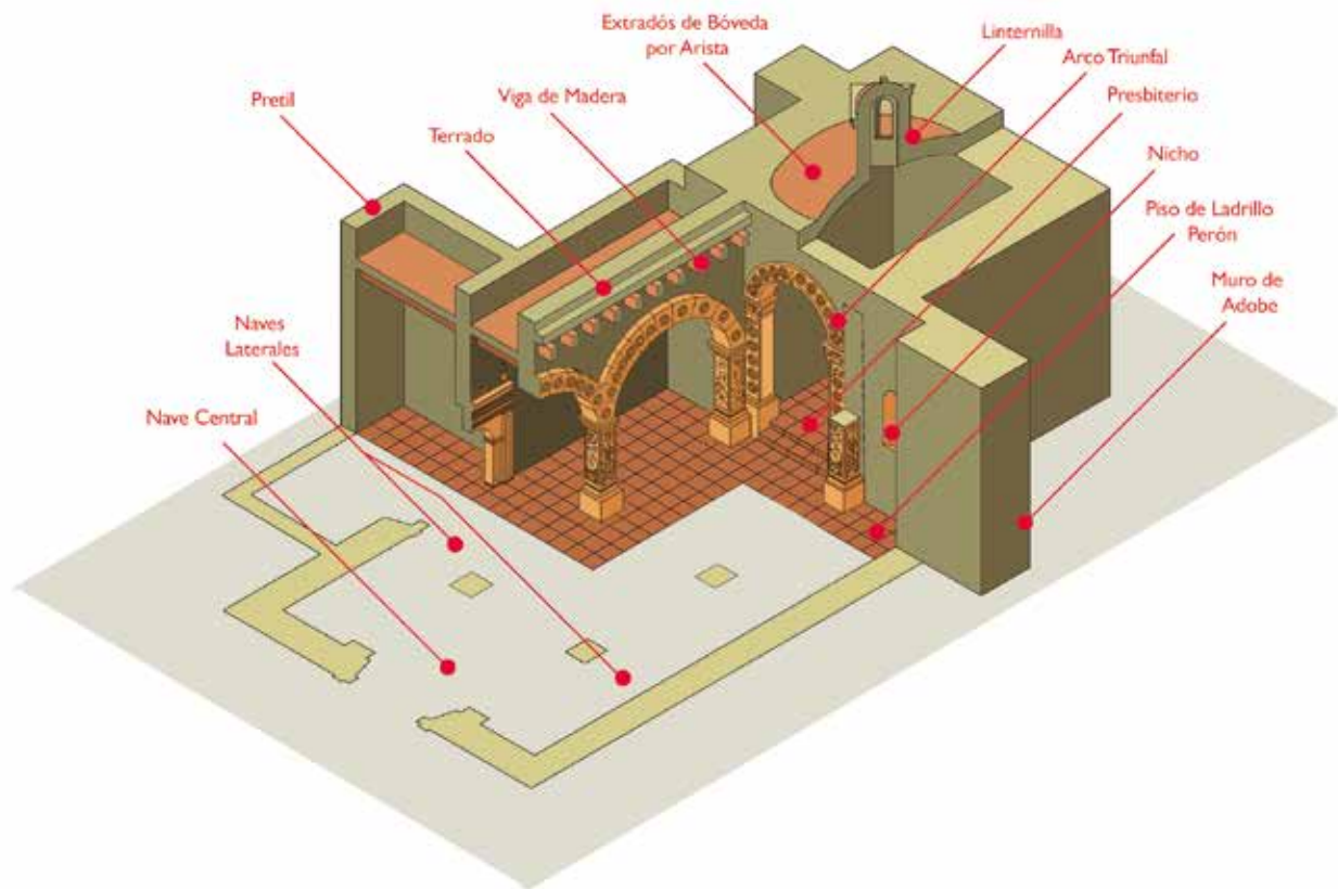
Figura 130. Detalles constructivos de la capilla de hospital de San Sebastián el Grande.
