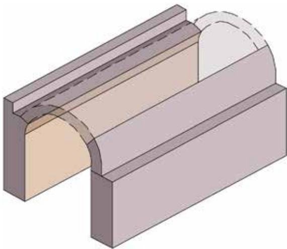
Figura 123. Bóveda de cañón corrido. Fuente: Elaboración propia, 2009.
