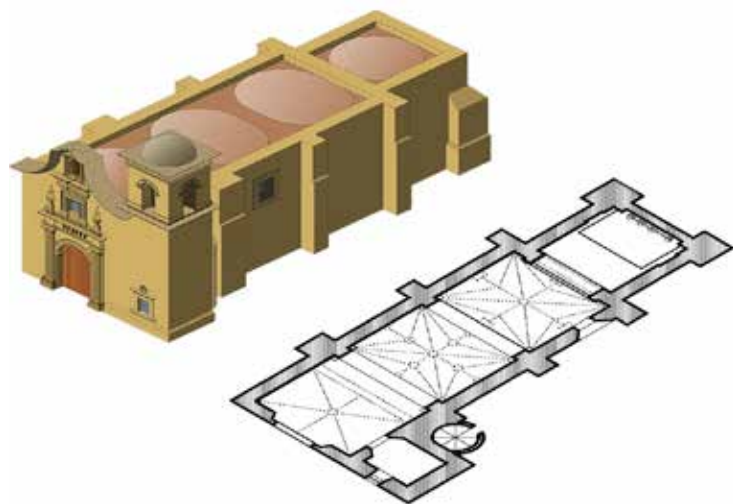
Figura 134. Dibujo y planta de Huentitán.
