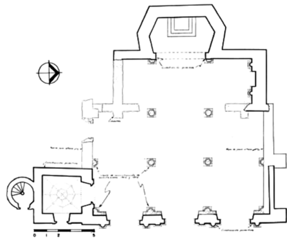
Figura 102. Planta arquitectónica del estado ruinoso en que se encontraba la capilla de Santa Cruz de las Flores. Dibujo: Juan Benito Artigas.
