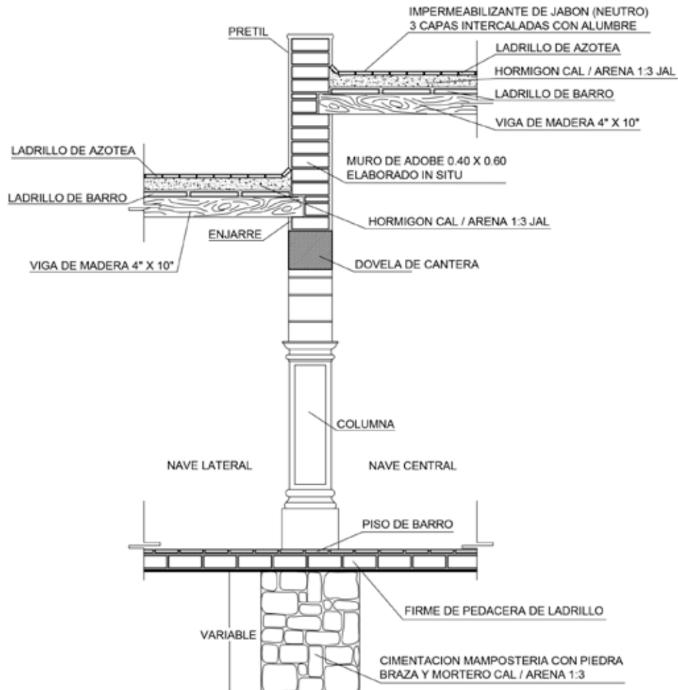
Figura 132. Detalle constructivo entre la nave central y lateral de la capilla de hospital de San Sebastián el Grande. Fuente: Elaboración propia, 2008.
