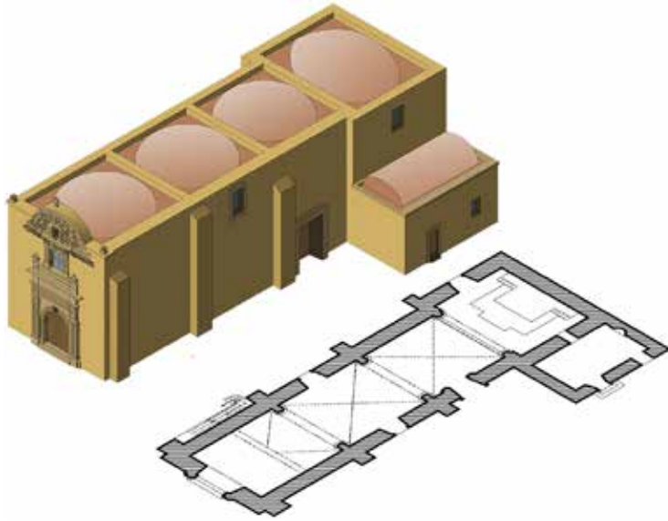
Figura 135. Dibujo y planta de Tlajomulco. Fuente: Elaboración propia, 2008.
