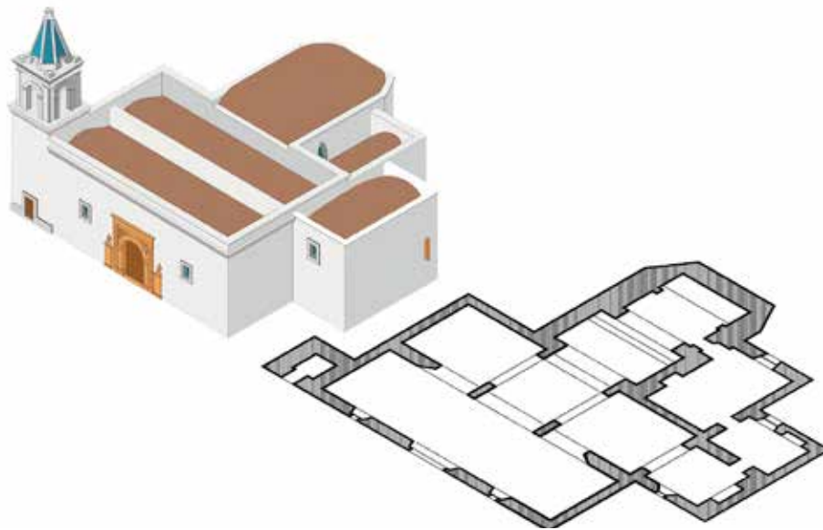
Figura 136. Dibujo y planta de San Agustín. Fuente: Elaboración propia, 2008.
