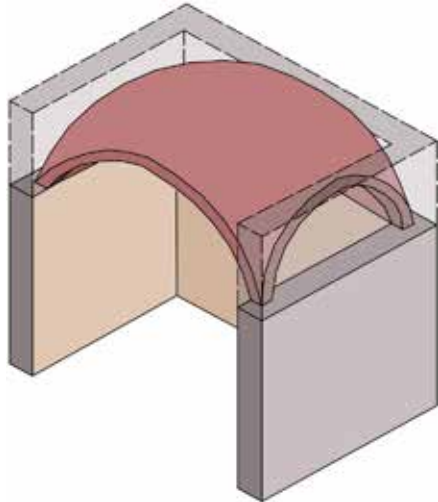
Figura 122. Proceso constructivo de la bóveda por arista. Fuente: Elaboración propia, 2009.
