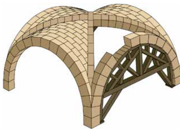
Figura 120. Proceso constructivo de la bóveda por arista. Fuente: Elaboración propia, 2009.
