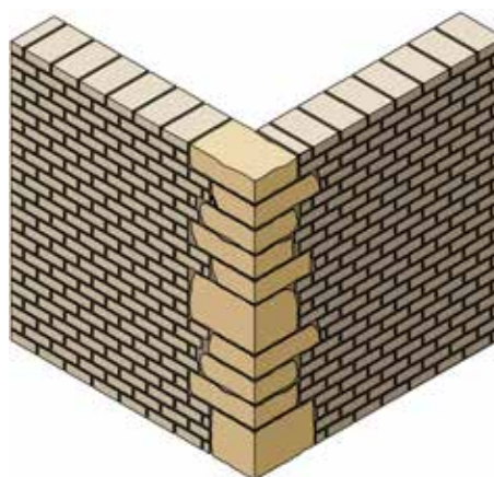
Figura 118. Traslape de piezas de cantera, como refuerzo estructural en aristas de muros de adobe. Fuente: Elaboración propia, 2009.
