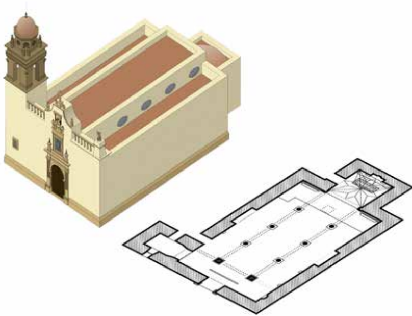
Figura 113. Vista isométrica con planta de la Capilla de San Andrés. Fuente: Elaboración propia, 2016.
