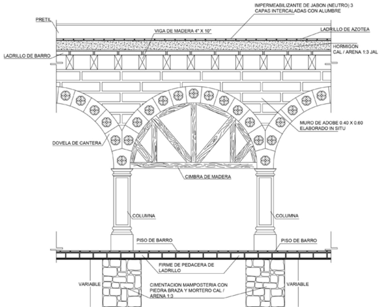
Figura 131. Detalles constructivos: división de la nave central y lateral de la capilla de hospital de San Sebastián el Grande. Fuente: Elaboración propia, 2008.
