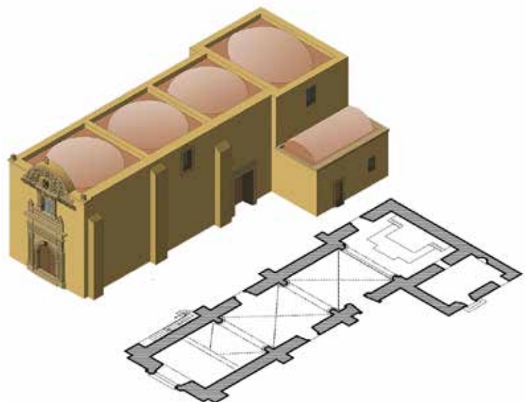
Figura 85. Vista isométrica con planta de la Capilla de Tlajomulco.
