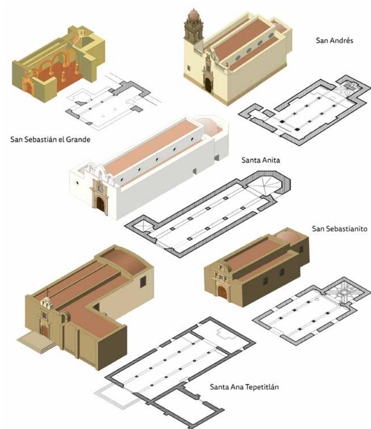
Figura 133. Dibujo de plantas de San Sebastián el Grande, San Andrés, Santa Anita, Santa Ana Tepetitlán y San Sebastianito. Fuente: Elaboración propia, 2016.
