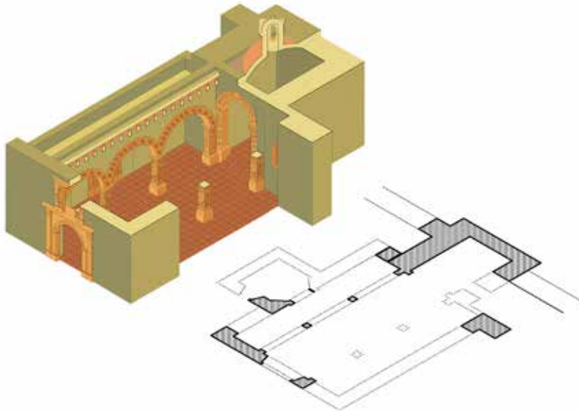
Figura 89. Vista isométrica con planta de la Capilla de San Sebastián El Grande. Fuente: Elaboración propia, 2016.
