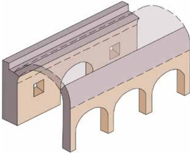
Figura 97. Bóveda de cañón sobre arcos en el primer tramo de la capilla de San Agustín. Fuente: Elaboración propia, 2008.
