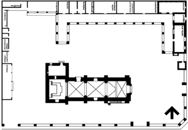
Figura 75. Planta arquitectónica actual del Hospital de la Purísima Concepción, Tlajomulco. Fuente: Elaboración propia, 2010.
