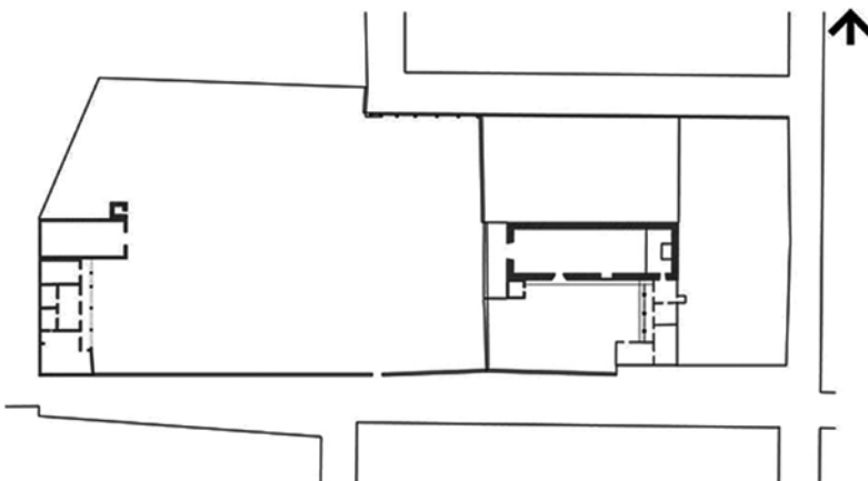
Figura 79. Planta arquitectónica del hospital de la Purísima Concepción, Ataco, Tapalpa, Jalisco. Fuente: Elaboración propia, 2010.
