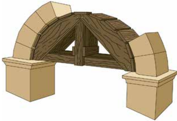
Figura 126. Detalle de cimbra de madera bajo arco de medio punto. Fuente: Elaboración propia, 2009.
