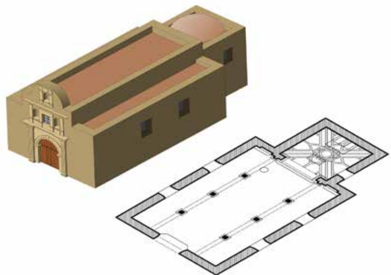
Figura 110. Vista isométrica con planta de la Capilla de San Sebastianito. Fuente: Elaboración propia, 2008.
